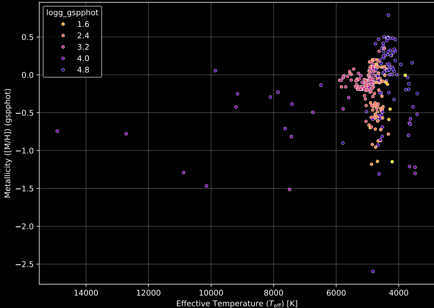
APOGEE DR17 Field: [169-24_btx] Stellar Population Parameters (n= 300)
